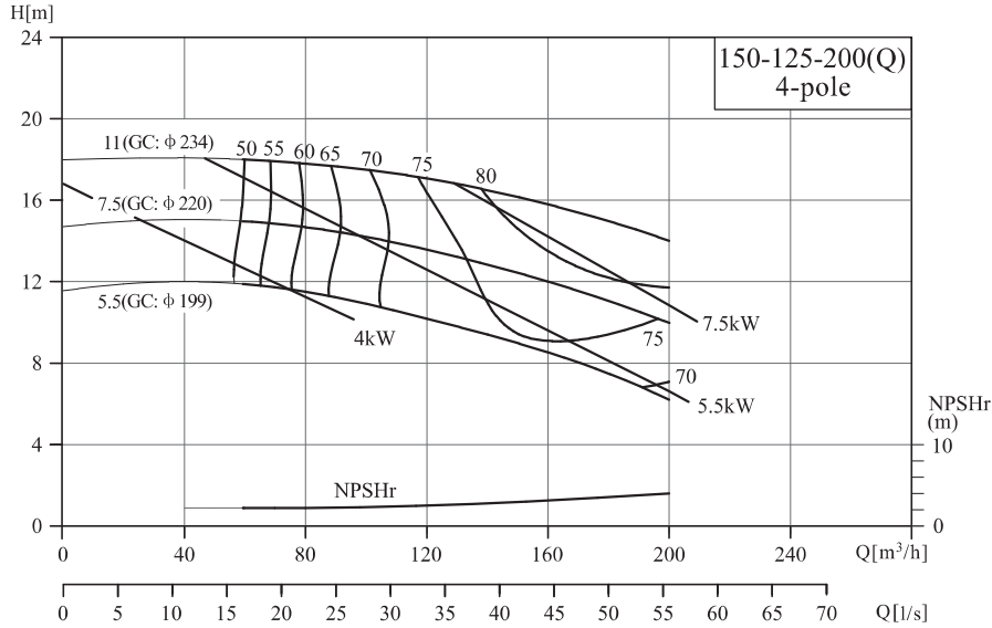
NIS150-125-200(Q)/150-125-200G
